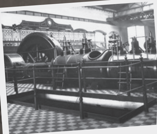
Blick ins Maschinenhaus, ca. 1901
